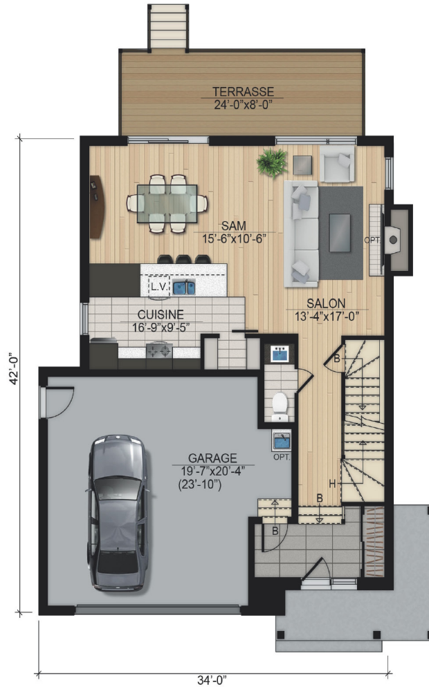
Rez-de-chaussée 899 pc
