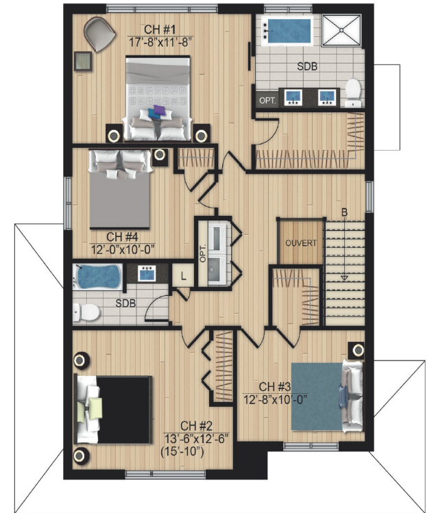
Étage 1177 pc
